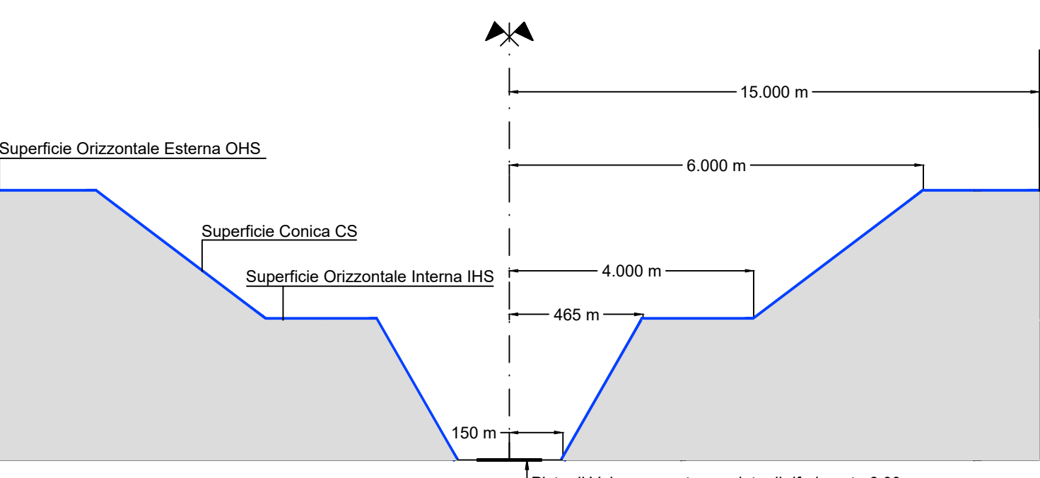
Sezione schematica delle superfici di limitazione degli ostacoli Art. 107 Vincolo militare e aeroportuale. (Scala di Vico con quota assoluta di riferimento 6.00 m.)
