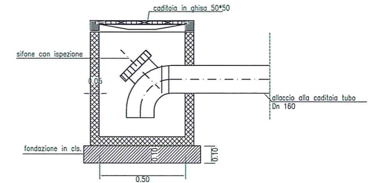
SEZIONE TIPO CUNETTA STRADALE scala 1:20
