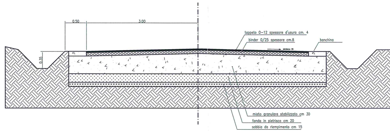
SEZIONE STRADALE TIPO scala 1:20
